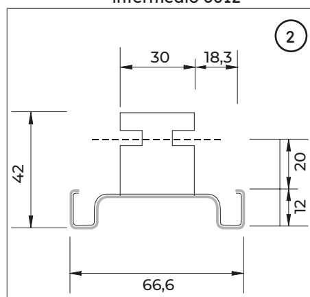
Perfil gola vertical intermedio 8012
